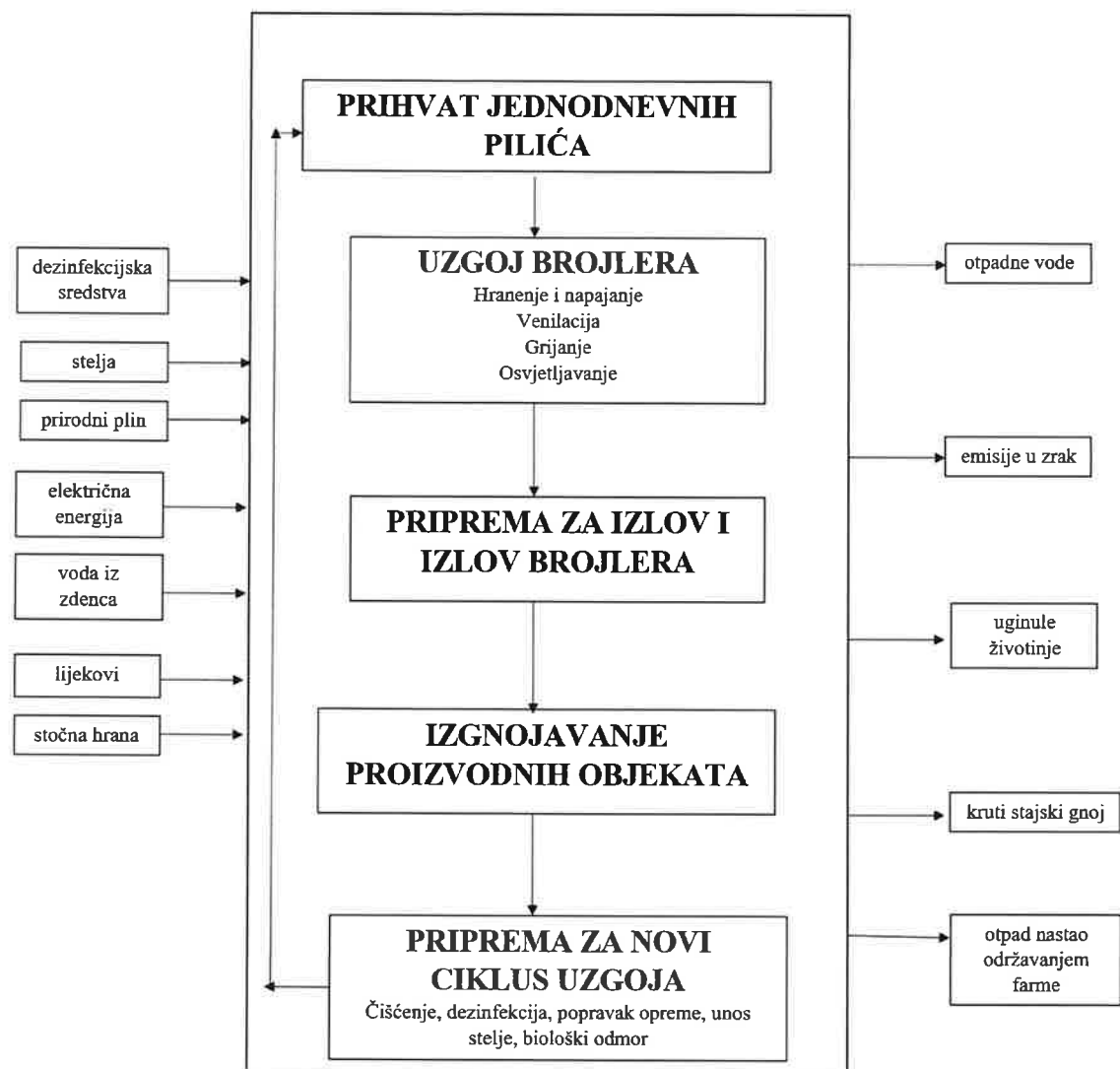
Prilog 2. Blok dijagram tehnološkog procesa na postojećem postrojenju za intenzivan uzgoj peradi Farma 17
